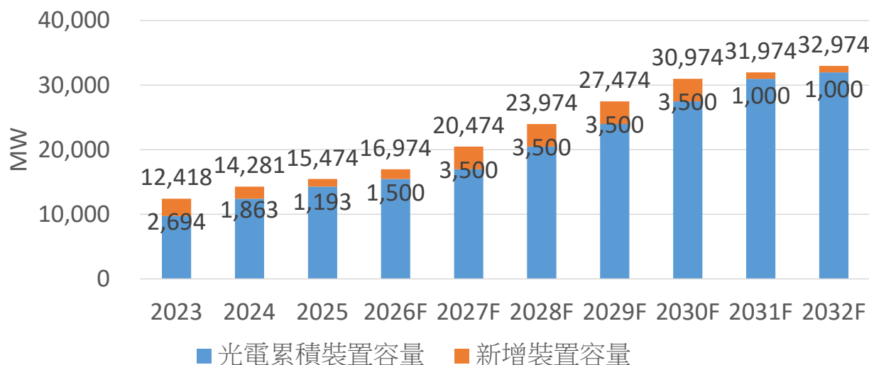
光電併網時程
