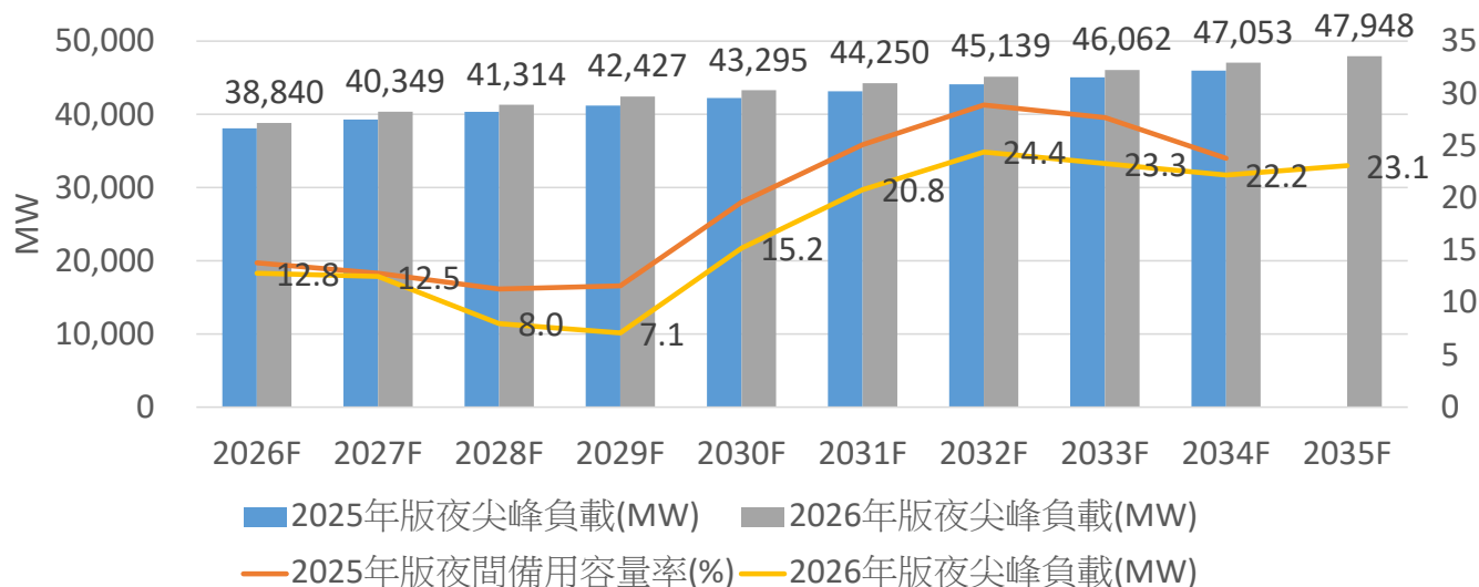
台灣2026~2035年夜間備用容量率
